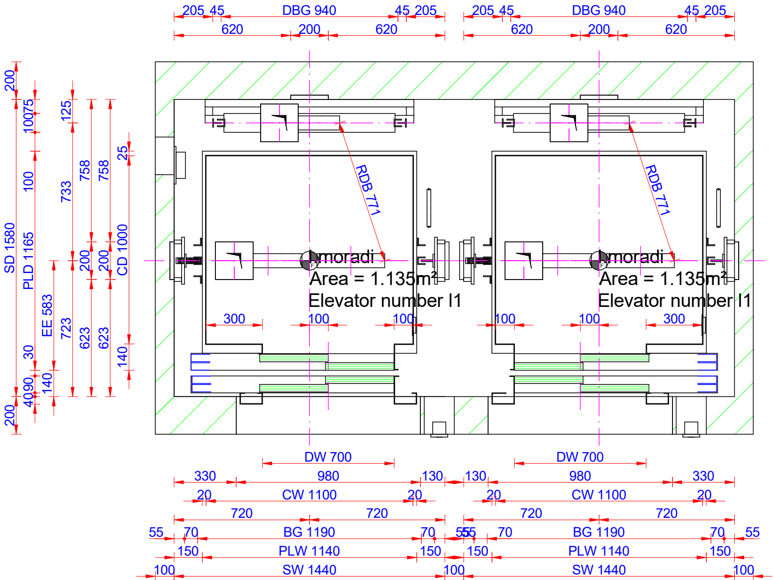
Plan Scale: 1:20
